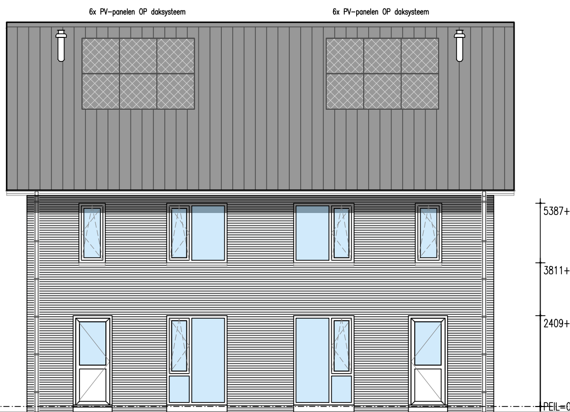
Achtergevel
