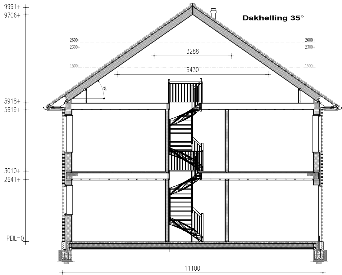
DOORSNEDE
